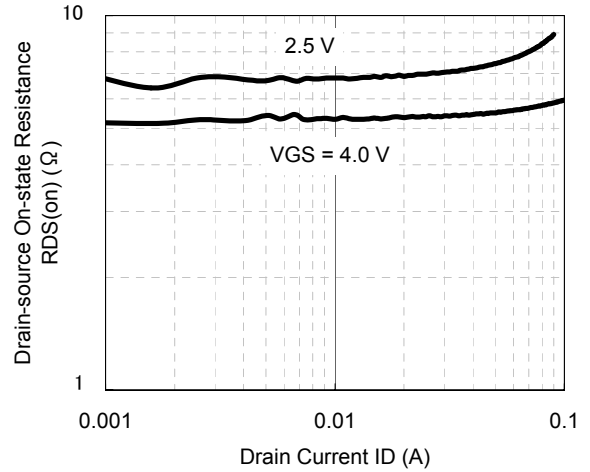
RDS(on) - ID
