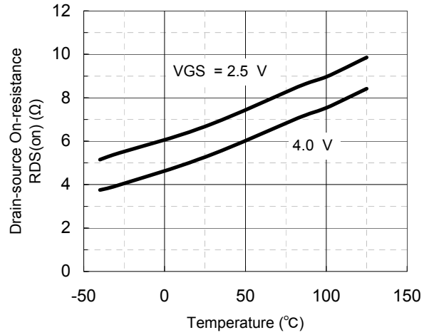
RDS(on) - Ta
