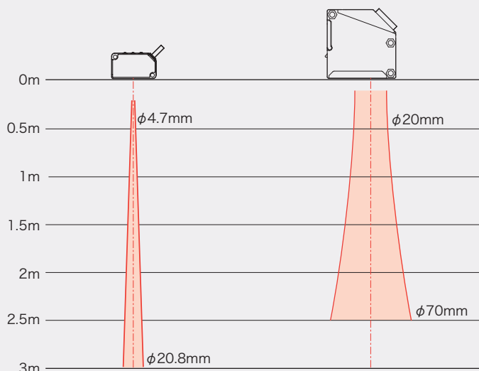
当社距離設定反射型ビームセンサ EQ-500シリーズ
