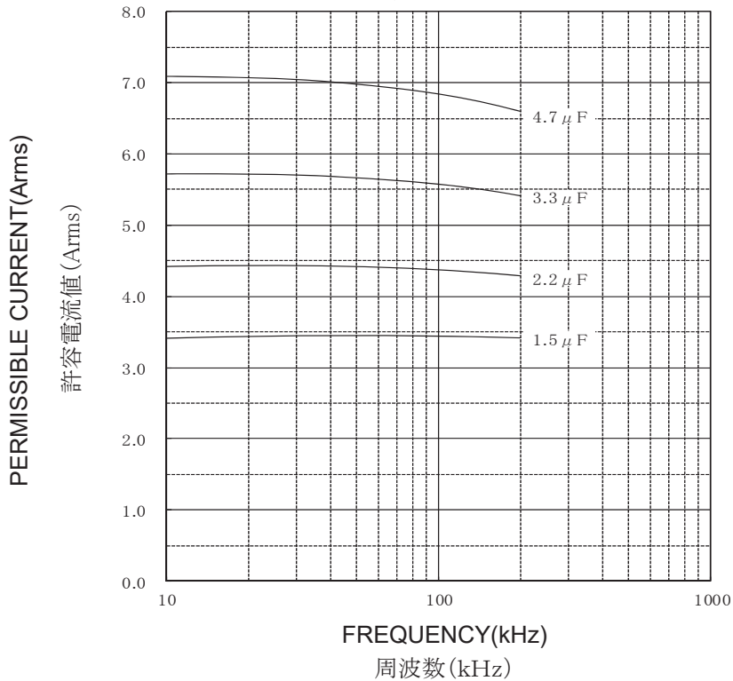
Lead Spacing 27.5mm リードピッチ 27.5mm
