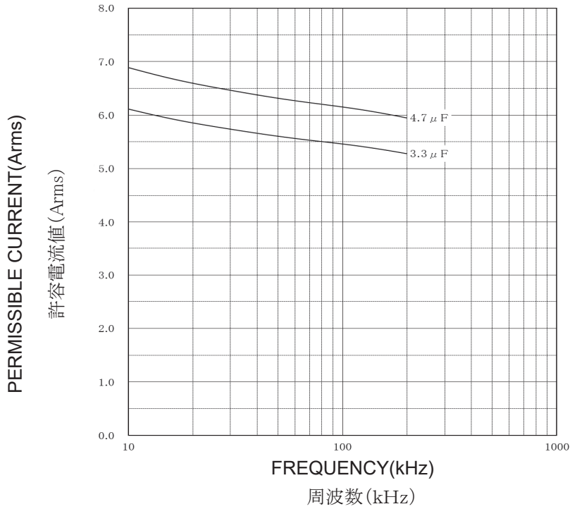
Lead Spacing 22.5mm リードピッチ 22.5mm
