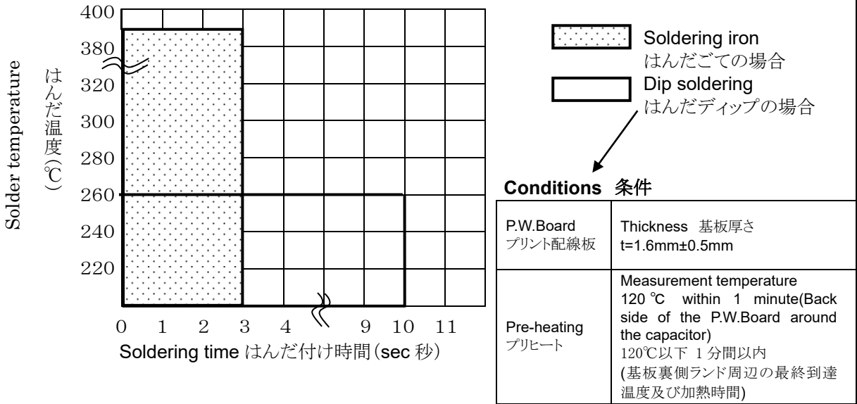
Fig.5 図-5 Recommend soldering condition 許容はんだ付け条件
