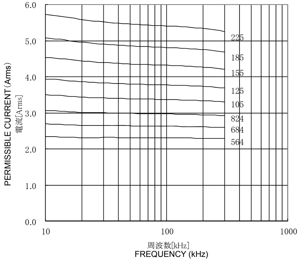
周波数別許容電流値(続き)
