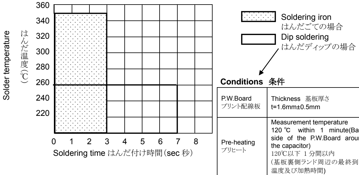
Fig.5 図-5 Recommend soldering condition 許容はんだ付け条件
