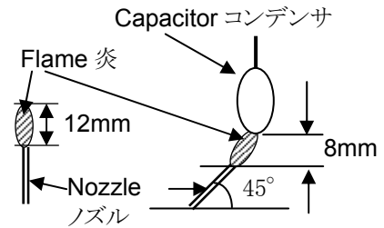
Schematic(概略図)
