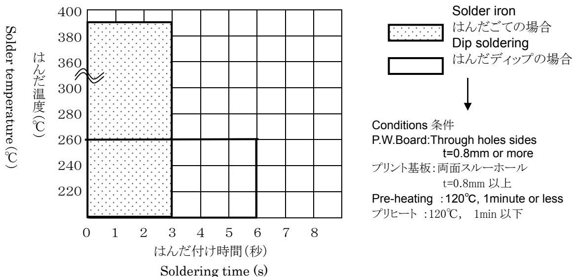
図-1 許容はんだ付け条件
