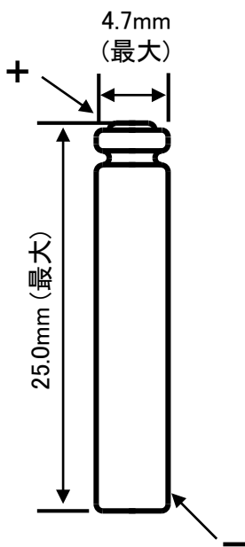
外形寸法図
