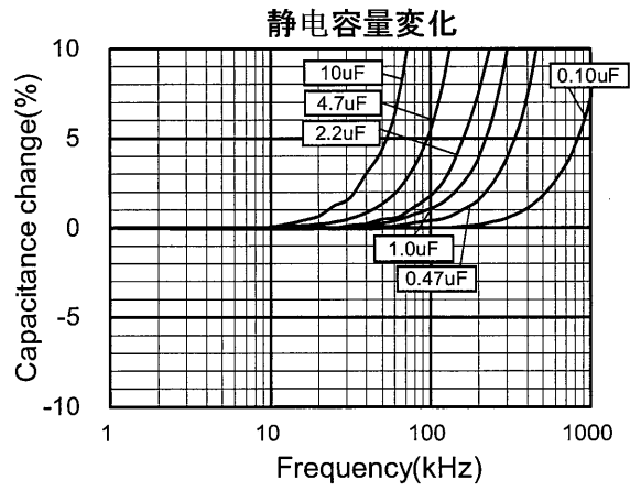
频率特性
