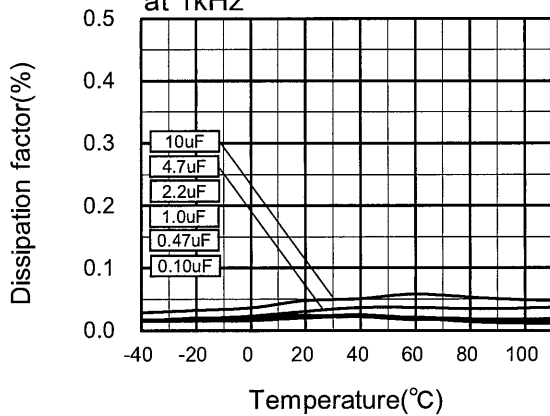
介质损耗因数变化
