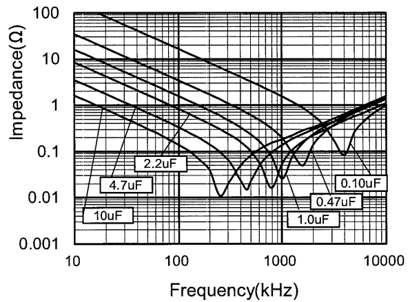
阻抗特性
