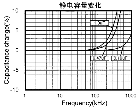
频率特性
