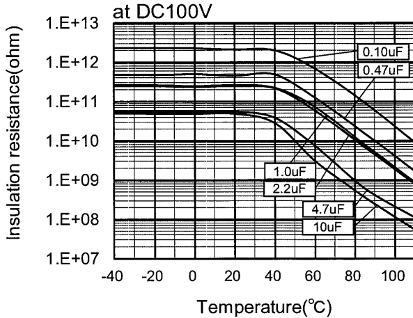
绝缘电阻变化
