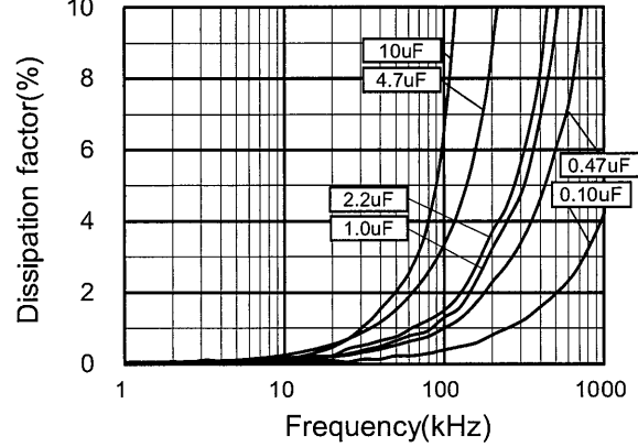
介质损耗因数变化
