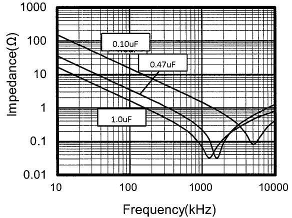
阻抗特性
