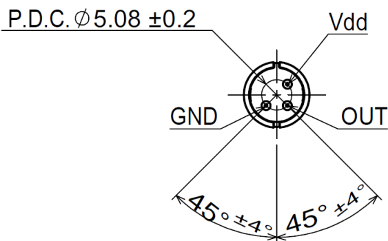
底面図
