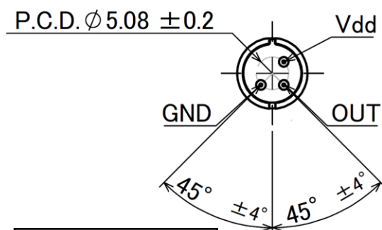
底面図
