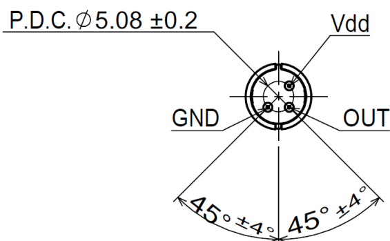
底面図
