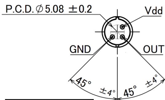
底面図
