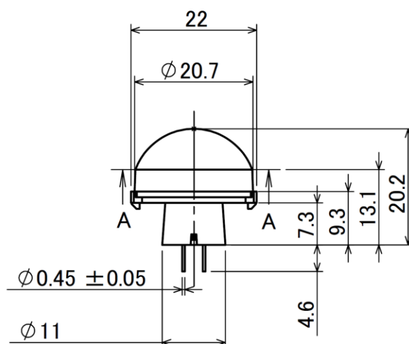
側面図
