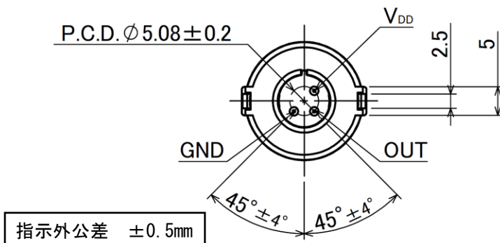
底面図
