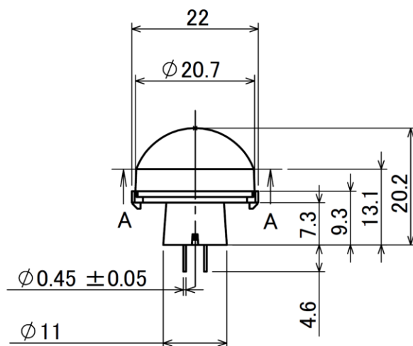
側面図
