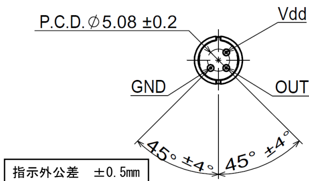
底面図
