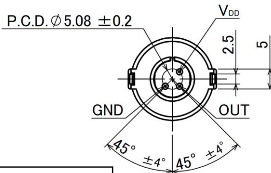
底面図
