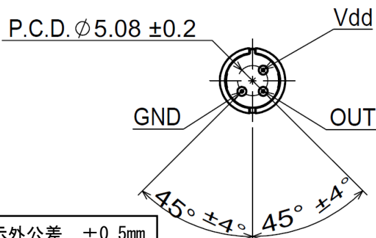
底面図
