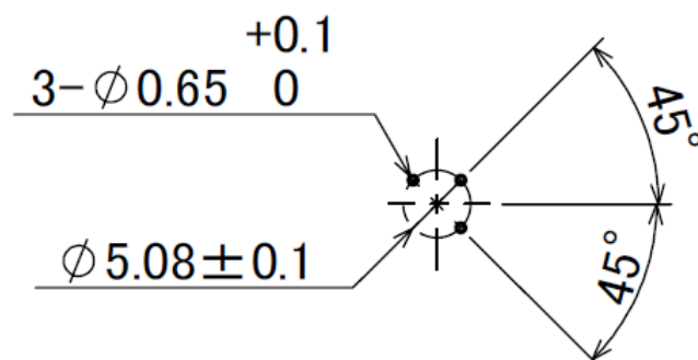
プリント基板推奨加工図
