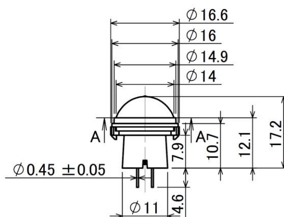
側面図
