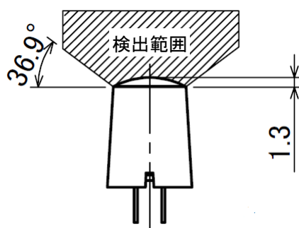
推奨穴加工寸法
