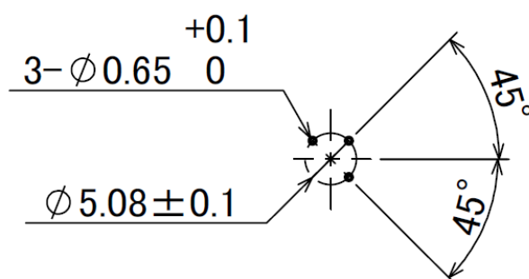
プリント板推奨加工図
