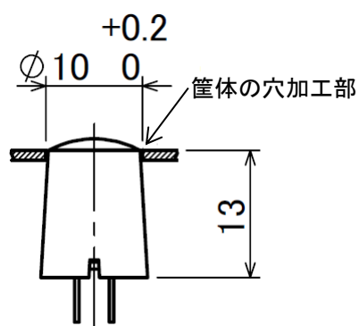
推奨穴加工寸法
