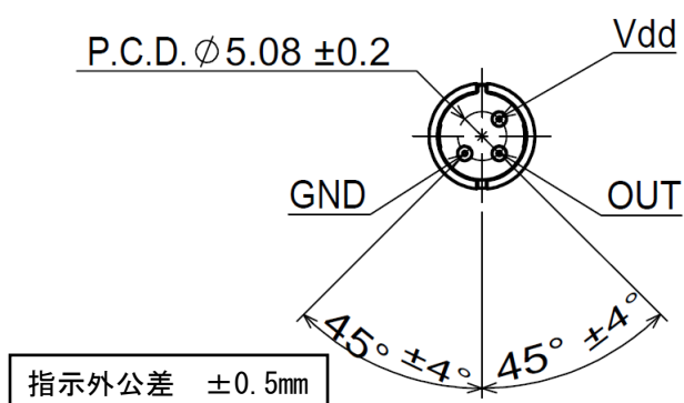
底面図
