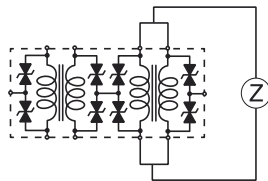
(A) 共模
