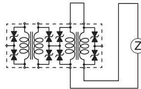
(B) 差模
