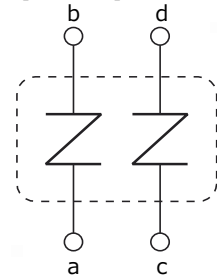
[电路构成]
