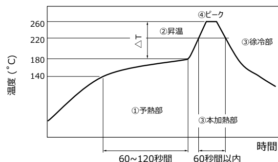
リフローはんだ付け推奨プロファイル（例）
