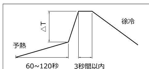
はんだこて付け推奨プロファイル（例）
