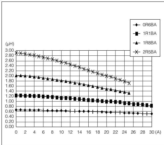
直流重畳特性
