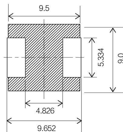
PCC-M1040M-LP 系列 (ETQP4M1R0KVC)
