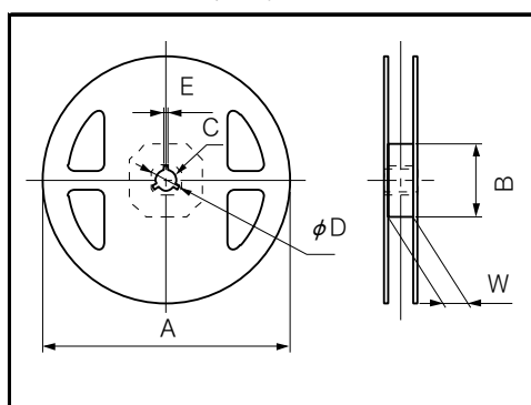
标准卷盘尺寸
