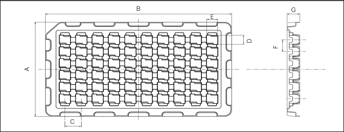
硬质泡沫塑料托盘 尺寸
