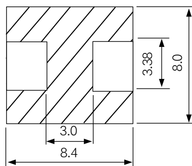
PCC-M0750M-LL 系列 (ETQP5M□□□CVM)
