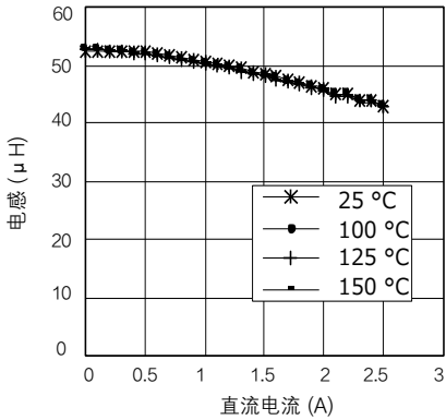
(表1): 直流重叠特性及温度特性 ETQP5M470YFM (参考特性)
