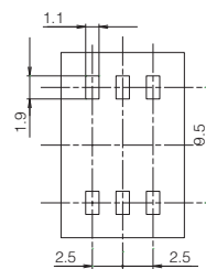
印刷电路板推荐加工图 (TOP VIEW)
