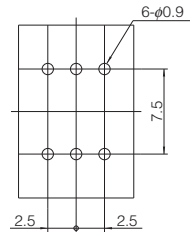
印刷电路板推荐加工图 (BOTTOM VIEW)
