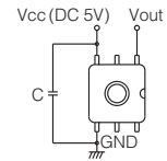
端子连接图
