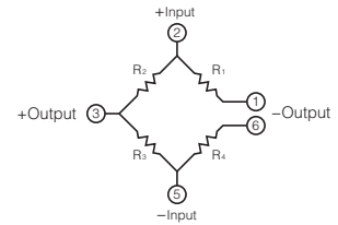
端子连接图
