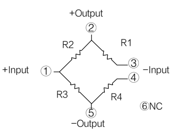
端子连接图
