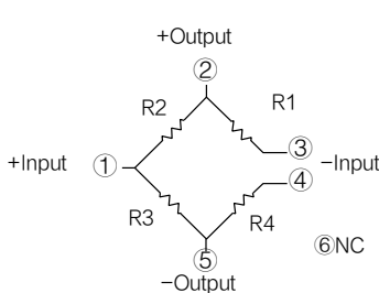
端子连接图
