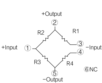
端子连接图
