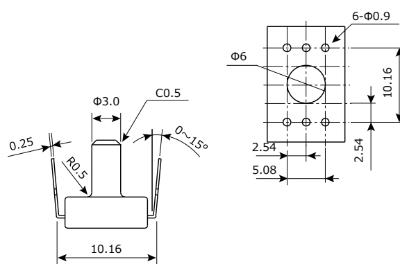
プリント板推奨加工図 (TOP VIEW)
