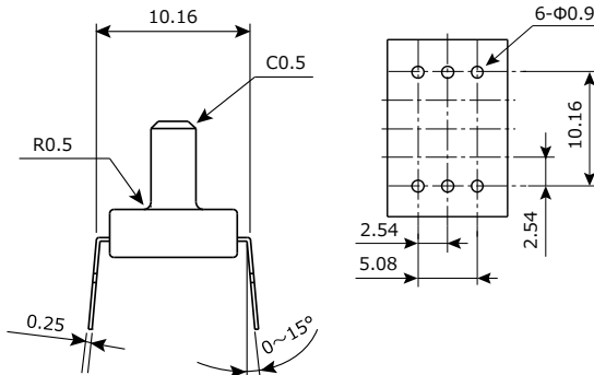
プリント板推奨加工図 (BOTTOM VIEW)
