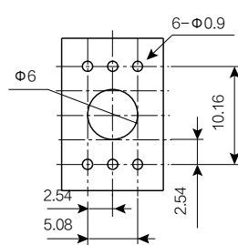
印刷电路板推荐加工图 (BOTTOM VIEW)
