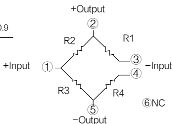
端子连接图
