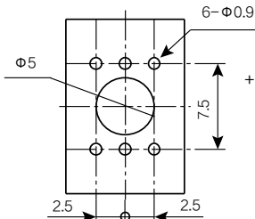
印刷电路板推荐加工图 (BOTTOM VIEW)
