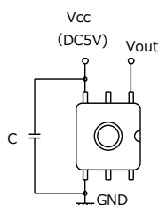
端子接続図
