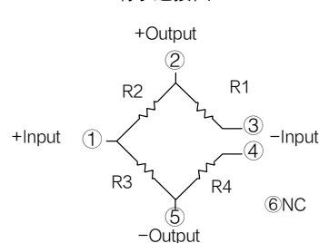
端子连接图
