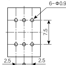
印刷电路板推荐加工图 (BOTTOM VIEW)
