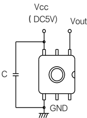
端子连接图
