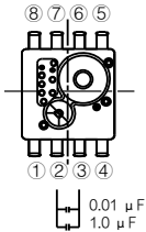
端子连接图
