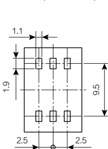
印刷电路板推荐加工图 (TOP VIEW)
