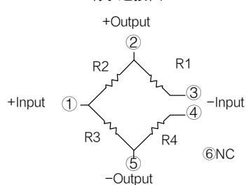
端子连接图
