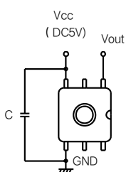
端子连接图
