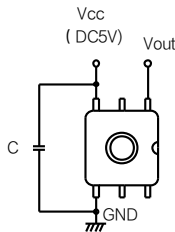
端子连接图
