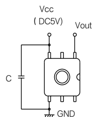
端子连接图
