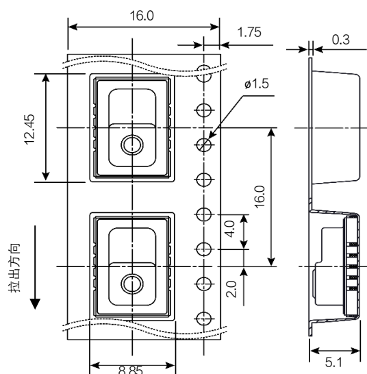
盘装形状及尺寸 (Typ.)
