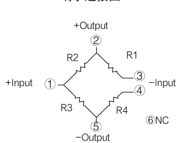
端子连接图
