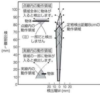
1.-(1) 薄型ショートタイプ (AMA1□□□□□□) ショートタイプ (AMBA1□□□□□□)
