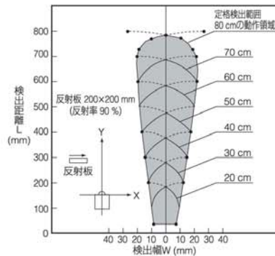
1.-(2) ミドルタイプ (AMBA2□□□□□□)
