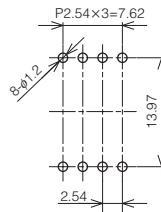
プリント板推奨加工図
