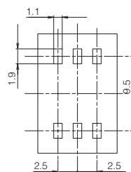
プリント板推奨加工図 (TOP VIEW)
