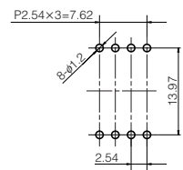
プリント板推奨加工図
