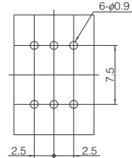
プリント板推奨加工図 (TOP VIEW)
