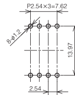
プリント板推奨加工図
