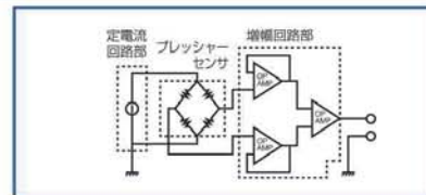
使用回路図 (例)
