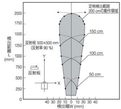
1.-(3) ロングタイプ (AMBA3□□□□□□)
