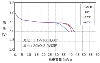
■ 放电特性
