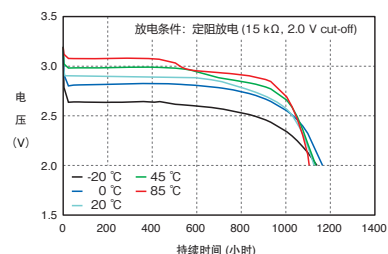
■ 放电温度特性(CR2032A示例)
