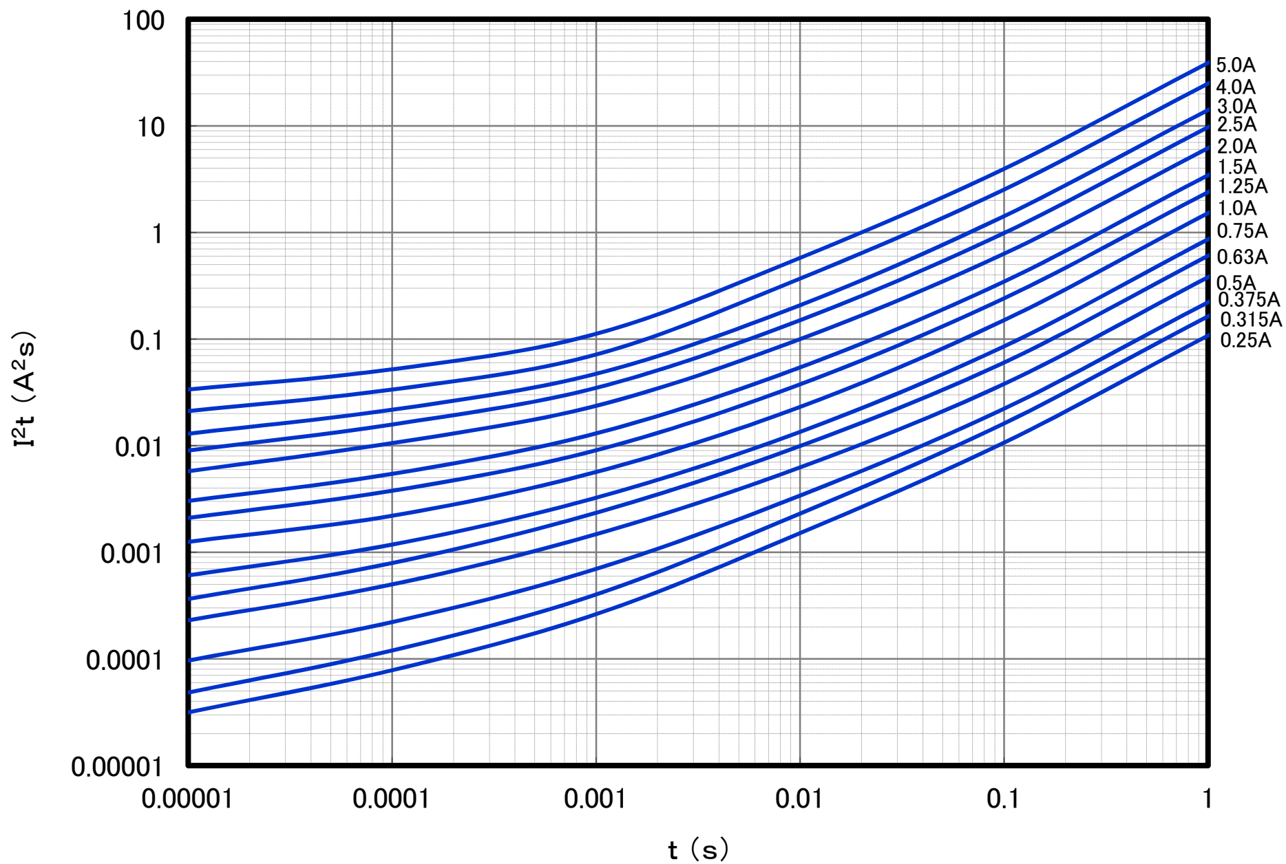
ERBRD系列 I^2t-t 特性 10万次耐受性曲线(25°C, 参考值)
